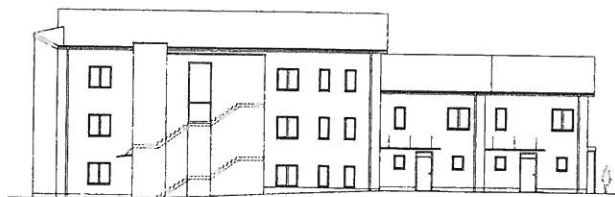
NORDANSICHT
