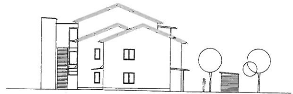
WESTANSICHT
